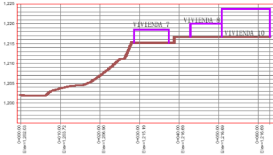
Figura 3. Sección crítica del área de estudio
