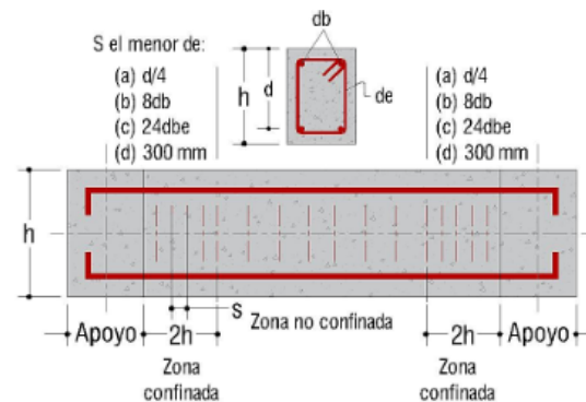
Figura 4. Estribos cerrados de confinamiento DMO
